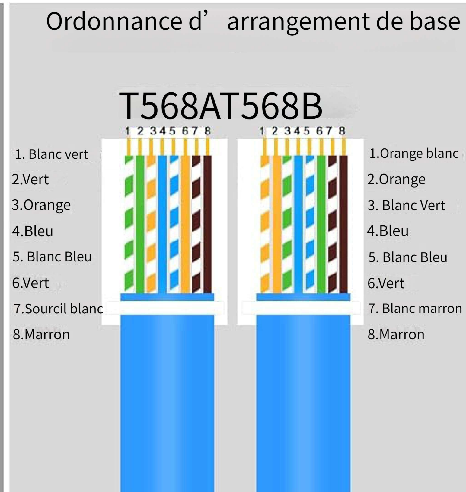
3. Organiser l'ordre des noyaux
