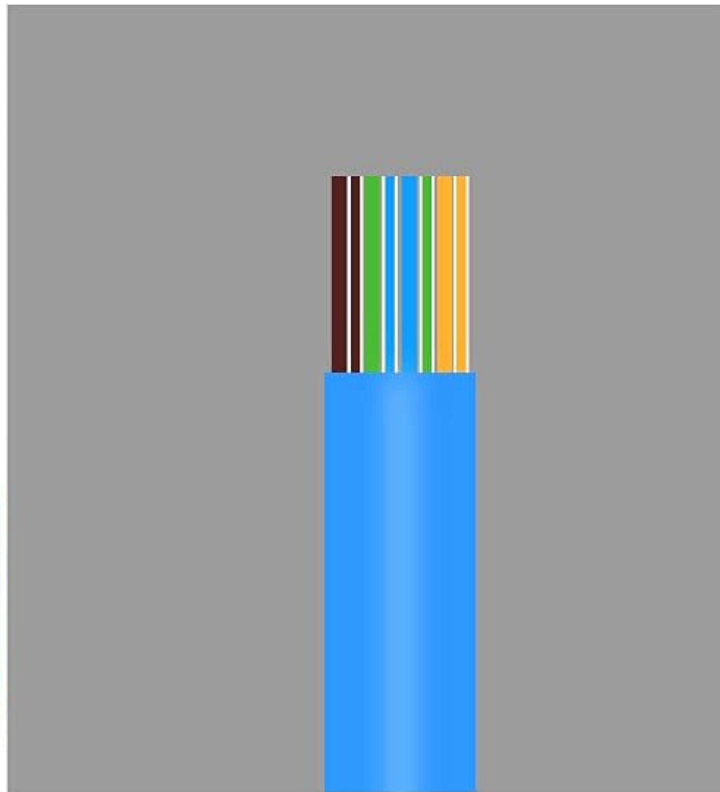
1.ワイヤーカッターを使用してシェルを切断します。 2.ネットワークケーブルシェルを取り出します。 3.芯の順番を整える ネットワークケーブルの
