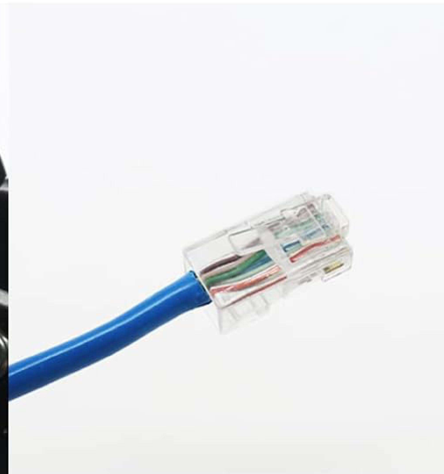
6.クリスタルの取り付け ヘッドとネットワークケーブルは、 完了しました
